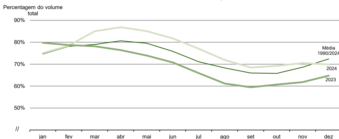
Armazenamento total nas principais albufeiras com aproveitamento hidroagrícola
