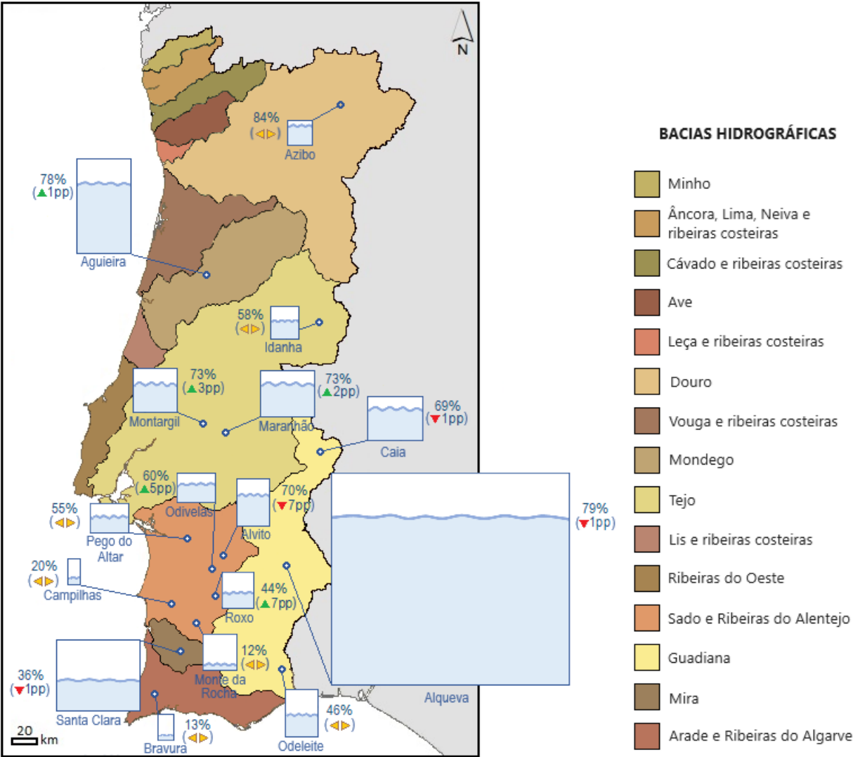
DISTRIBUIÇÃO ESPACIAL DO ÍNDICE DE SECA METEOROLÓGICA A 31 DE DEZEMBRO DE 2024 (COMPARAÇÃO COM 31 DE DEZEMBRO DE 2023 E 30 DE NOVEMBRO DE 2024)
